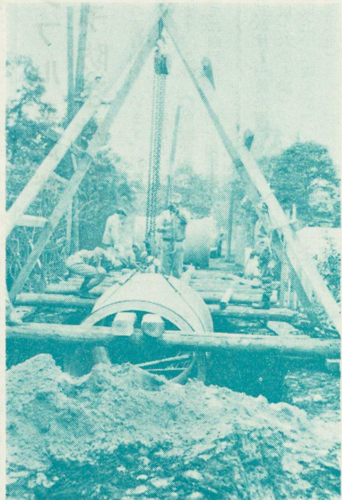
△ 昨年の和泉幹線下水道工事
